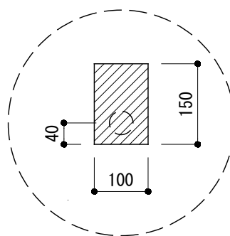
カウンター切込寸法
