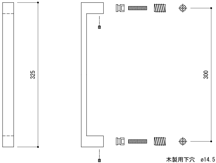
<切欠図>
