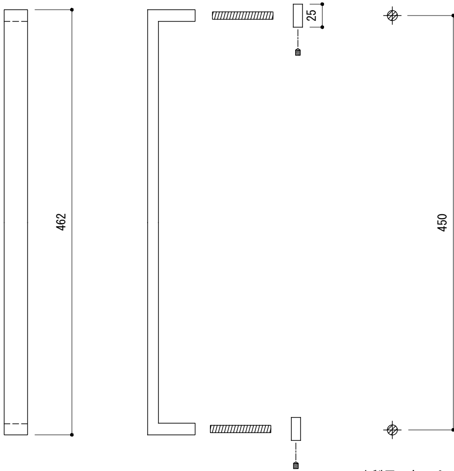
〈切欠図〉
