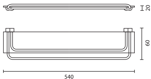
KUF74-4505 シェルフ
