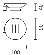
KUF74-4503 ソープディッシュ
