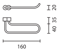
KUF74-4501 トイレトペーパーホルダー
