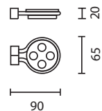
KUF74-4502 歯ブラシホルダー
