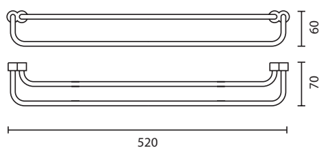
KUF74-4506 タオルバー
