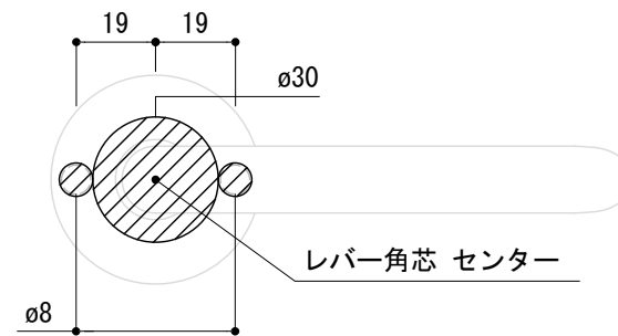
<切欠図>
