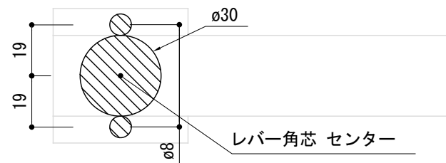
〈切欠図〉
