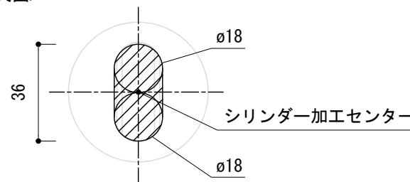
<切欠図>
