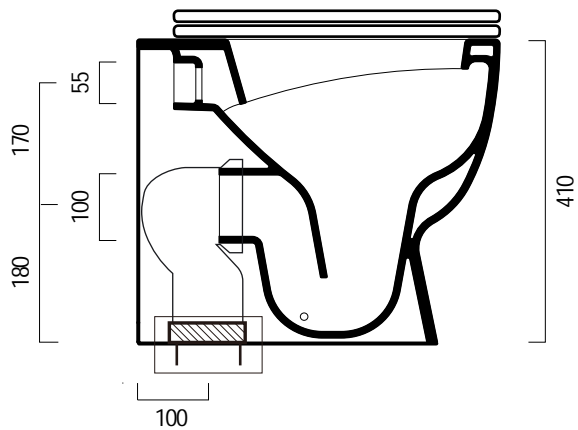
【排水部詳細図】
