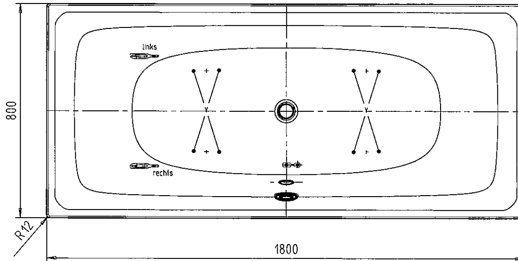
Position der Fußböcken nach 3D-Modell! (Fußmodell 5037)
