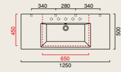
ZERODomino 125 lavabo washbasin waschtisch 125 x 50 cod. 125DO
