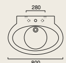
ZERO+ 80 lavabo washbasin waschtisch 80 x 56 cod. 80ZE
