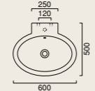
ZERO+ 60|2 lavabo washbasin waschtisch 60 x 50 cod. 6BZE
