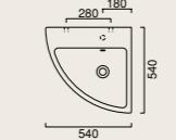
ZEROKono 54 lavabo washbasin waschtisch 54 x 54 cod. 54KO
