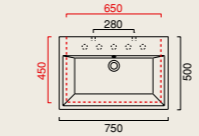
ZERO 75 lavabo washbasin waschtisch 75 x 50 cod. 75ZE
