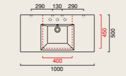
ZERODomino 100 lavabo washbasin waschtisch 100 x 50 cod. 10DO
