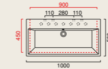
ZERO 100 lavabo washbasin waschtisch 100 x 50 cod. 10ZE
