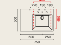
ZERODomino 75 Dx lavabo washbasin waschtisch 75 x 50 cod. 7DZE
