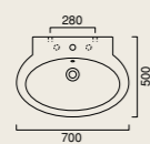
ZERO+ 70 lavabo washbasin waschtisch 70 x 50 cod. 70ZE
