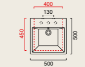
ZERO 50 lavabo washbasin waschtisch 50 x 50 cod. 5QZE
