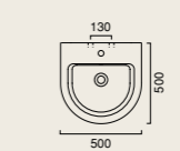
ZERO 50 tondo lavabo washbasin waschtisch 50 x 50 cod. 50ZN
