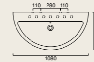
ZEROKono 108 lavabo washbasin waschtisch 108 x 54 cod. 10KO
