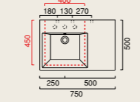
ZERODomino 75 Sx lavabo washbasin waschtisch 75 x 50 cod. 75ZE
