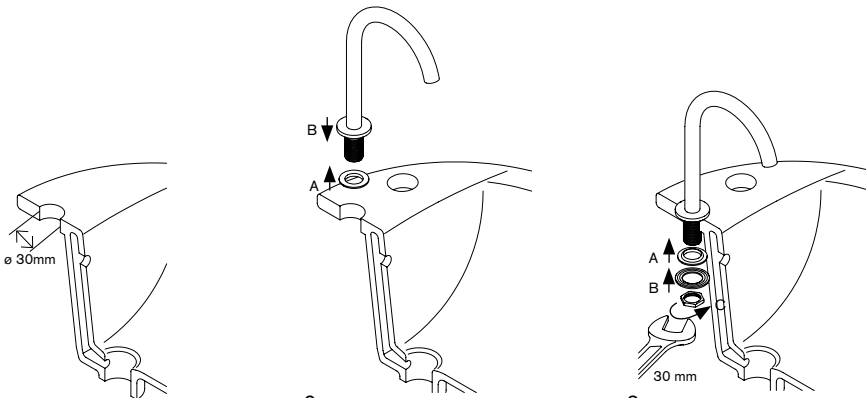
ART. B106WF Batteria lavabo / Washbasin / Lavabo 3 trous / Waschtischarmatur / Lavabo 3 piezas
