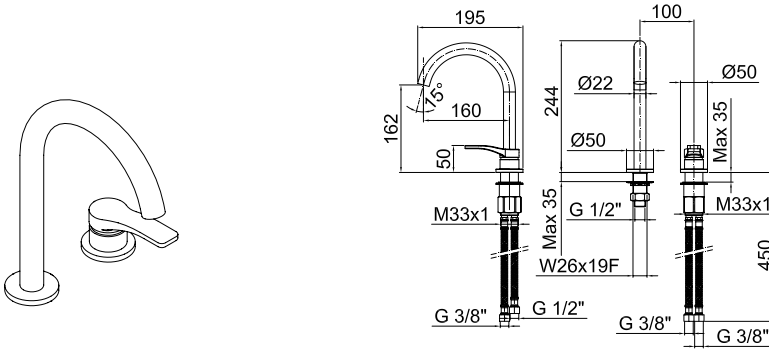
ART. B104WF Batteria lavabo / Washbasin / Lavabo 3 trous / Waschtischarmatur / Lavabo 3 piezas
