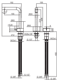
ART. A106WF Gruppo lavabo / Washbasin / Lavabo 1 trous / Waschtischarmatur / Lavabo
