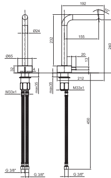
ART. A006WF Gruppo lavabo / Washbasin / Lavabo 1 trous / Waschtischarmatur / Lavabo
