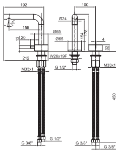
ART. A104WF Gruppo lavabo / Washbasin / Lavabo 1 trous / Waschtischarmatur / Lavabo
