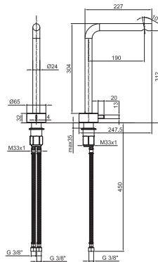
ART. A007WF Gruppo lavabo / Washbasin / Lavabo 1 trous / Waschtischarmatur / Lavabo
