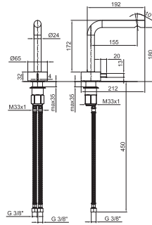
ART. A004WF Gruppo lavabo / Washbasin / Lavabo 1 trous / Waschtischarmatur / Lavabo
