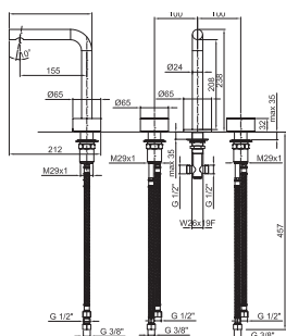
ART. A206WF Gruppo lavabo / Washbasin / Lavabo 1 trous / Waschtischarmatur / Lavabo
