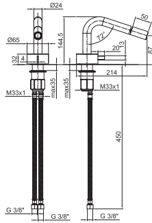
ART. A008WF Bidet monoforo / 1 hole bidet / Mélangeur bidet / Einlochbidet / Monobloc bidé
