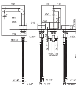
ART. A204WF Gruppo lavabo / Washbasin / Lavabo 1 trous / Waschtischarmatur / Lavabo
