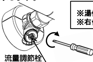
流量調節栓
