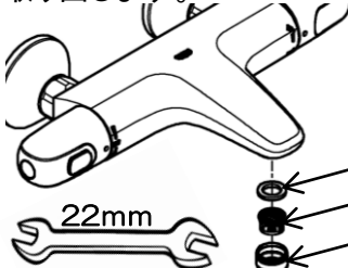
パッキン
