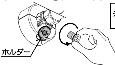
流量調節栓
