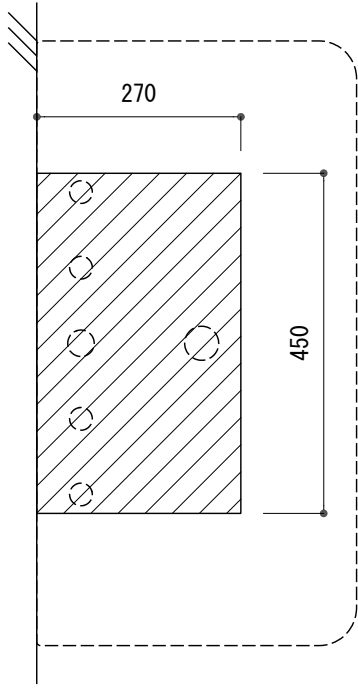
カウンター切込み寸法
