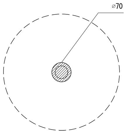
カウンター切込寸法
