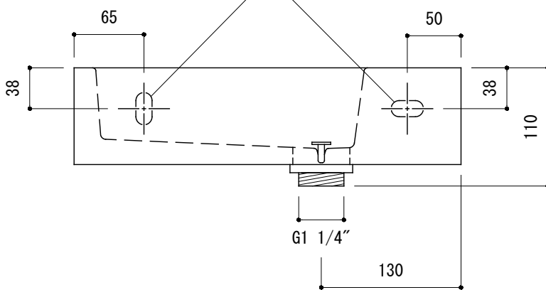
壁取付ボルト位置 (2ヶ所)
