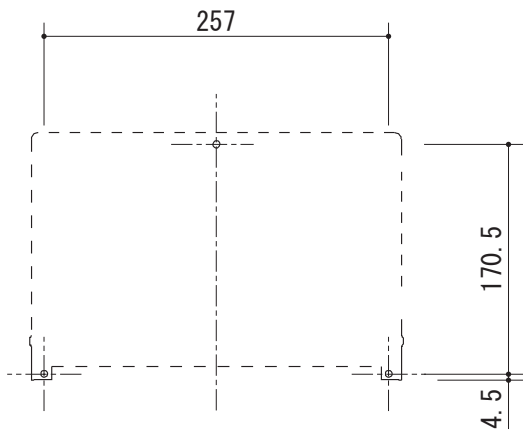
壁固定位置
