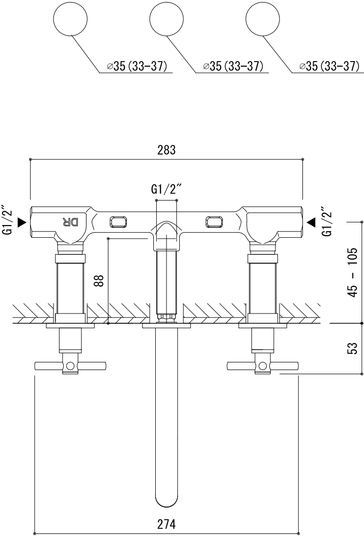
水栓取付穴
