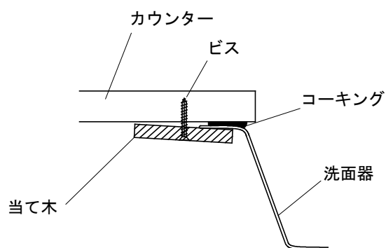
洗面器固定方法
