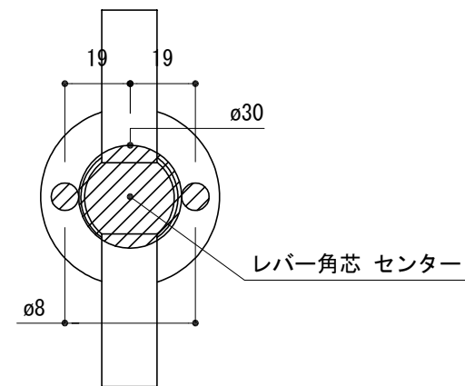
〈切欠図〉
