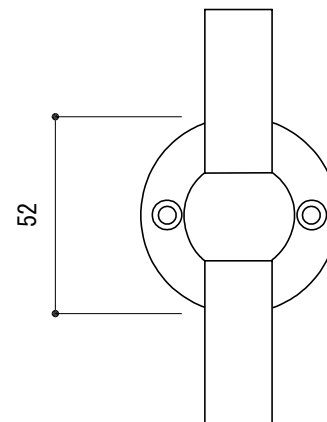
〈切欠図〉
