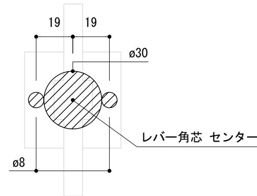
<切欠図>
