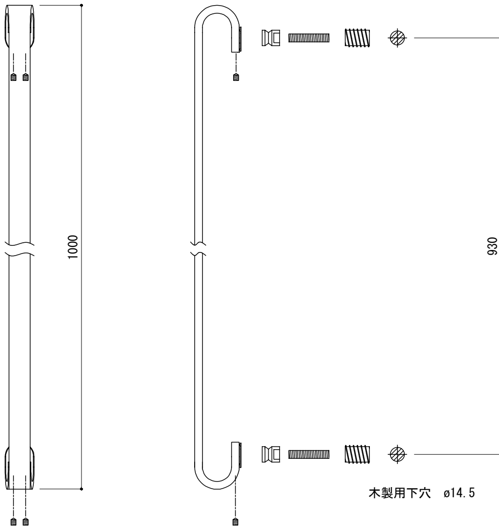
<切欠図>
