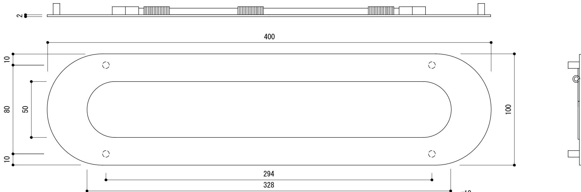
<切欠図>
