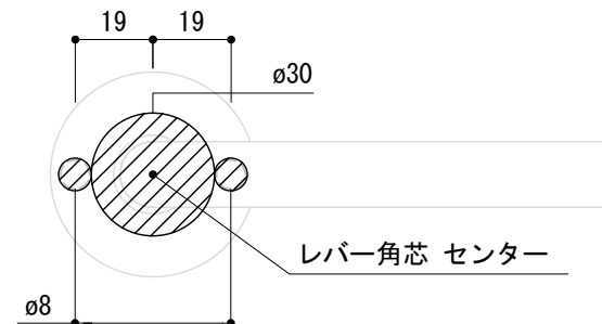
<切欠図>
