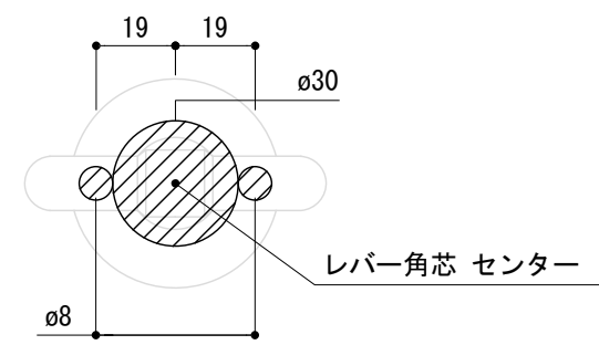
<切欠図>
