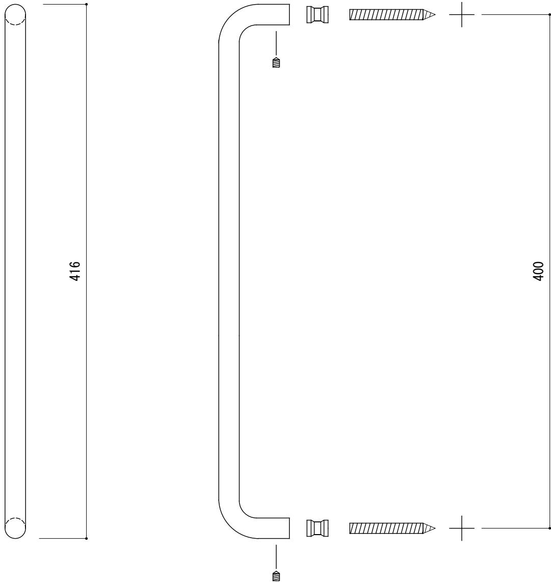
<切欠図>
