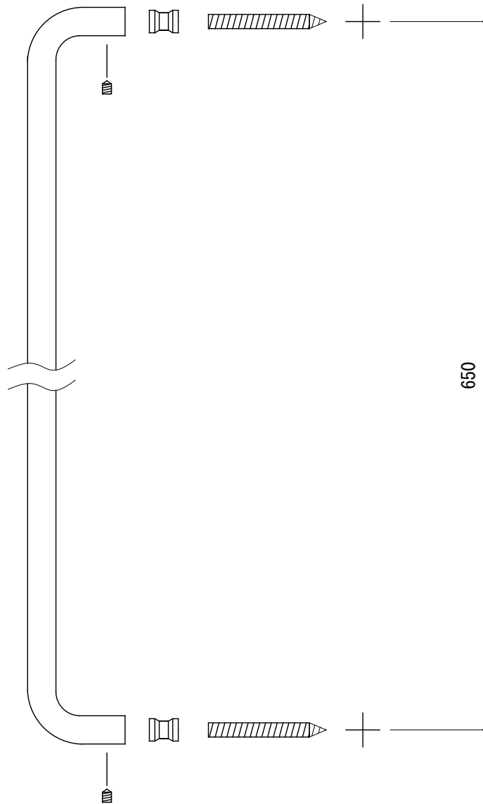
<切欠図>
