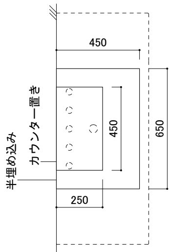
カウンター一切込寸法 (Not To Scale)
