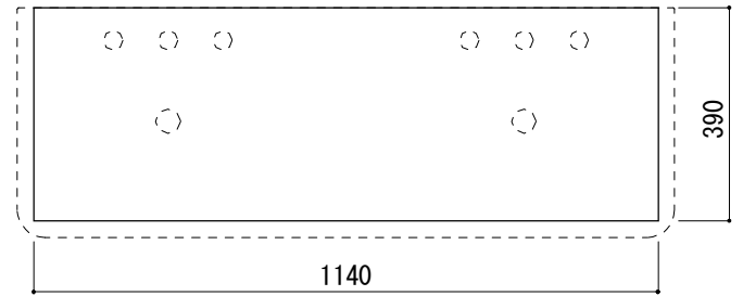
カウンター切込寸法
