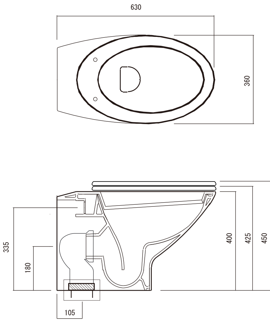
【排水部詳細図】
