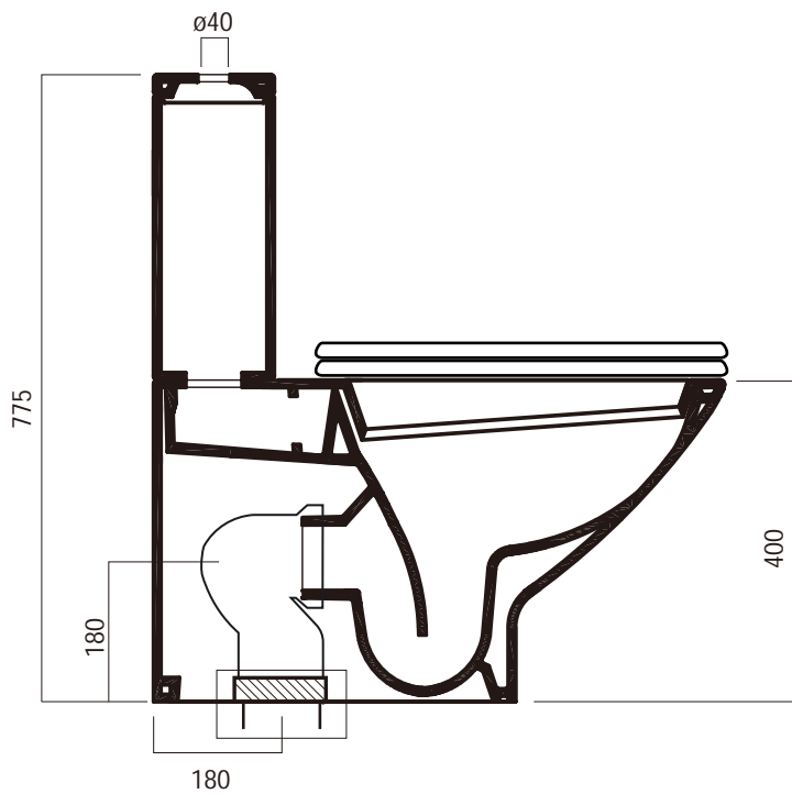
【排水部詳細図】
