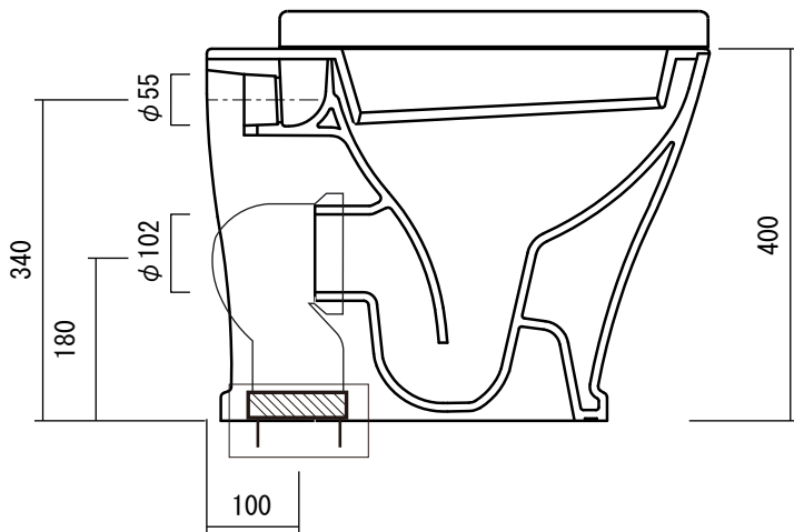
【排水部詳細図】
