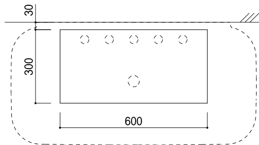
カウンター切込寸法
