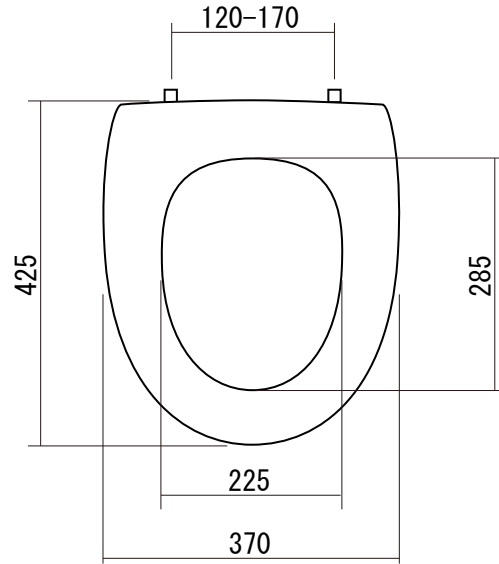
便座寸法
