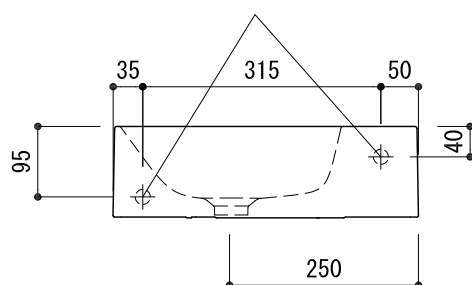
壁取付ボルト位置 (2ヶ所)
