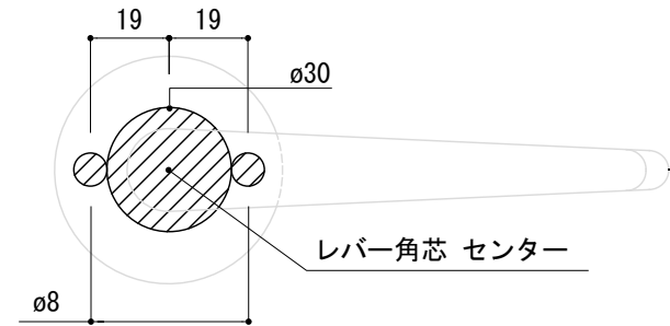
<切欠図>
