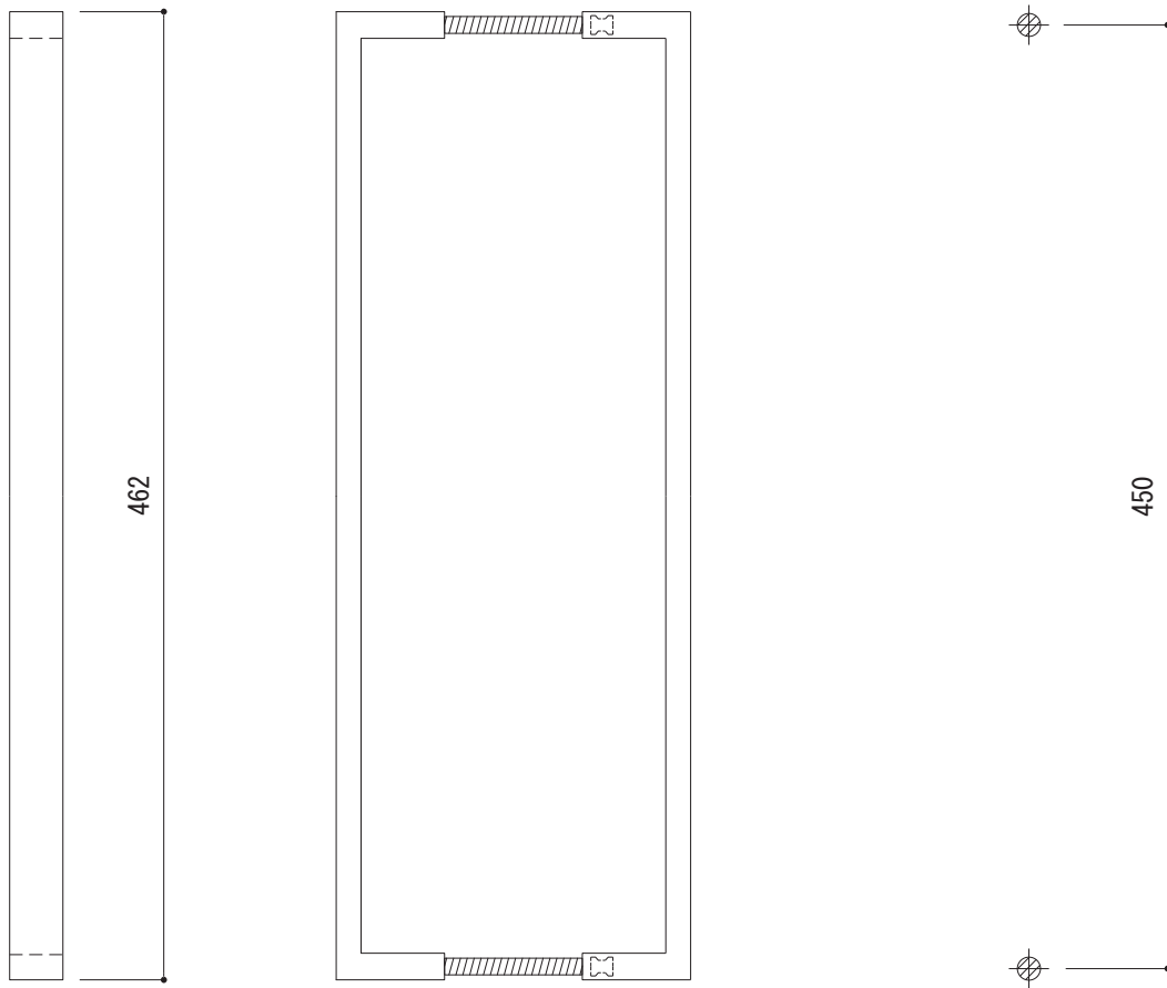
<切欠図>
