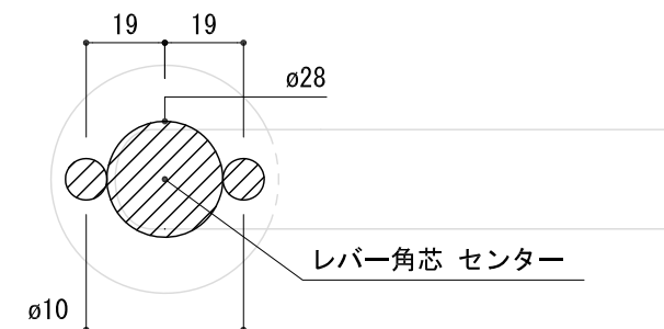
<切欠図>
