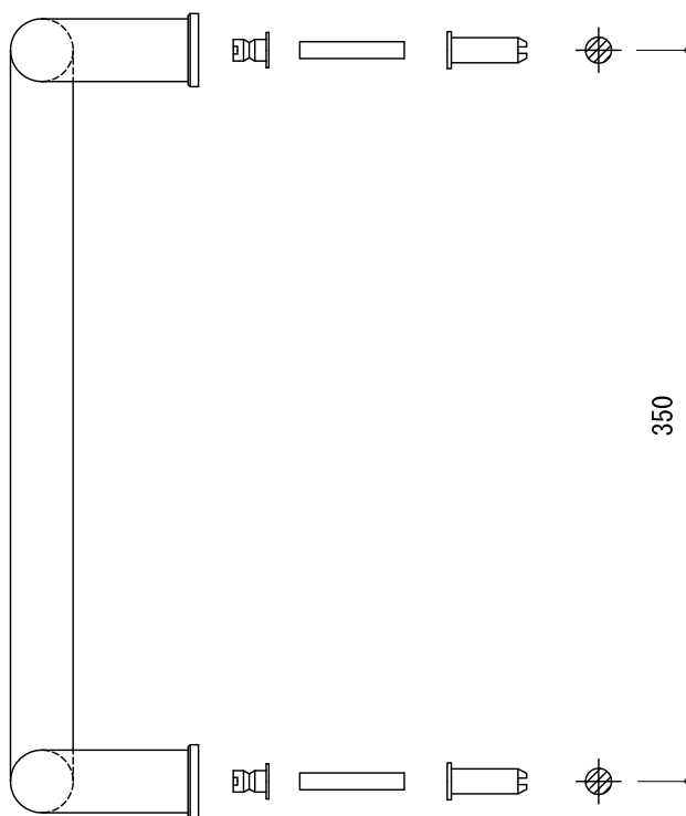
〈切欠図〉
