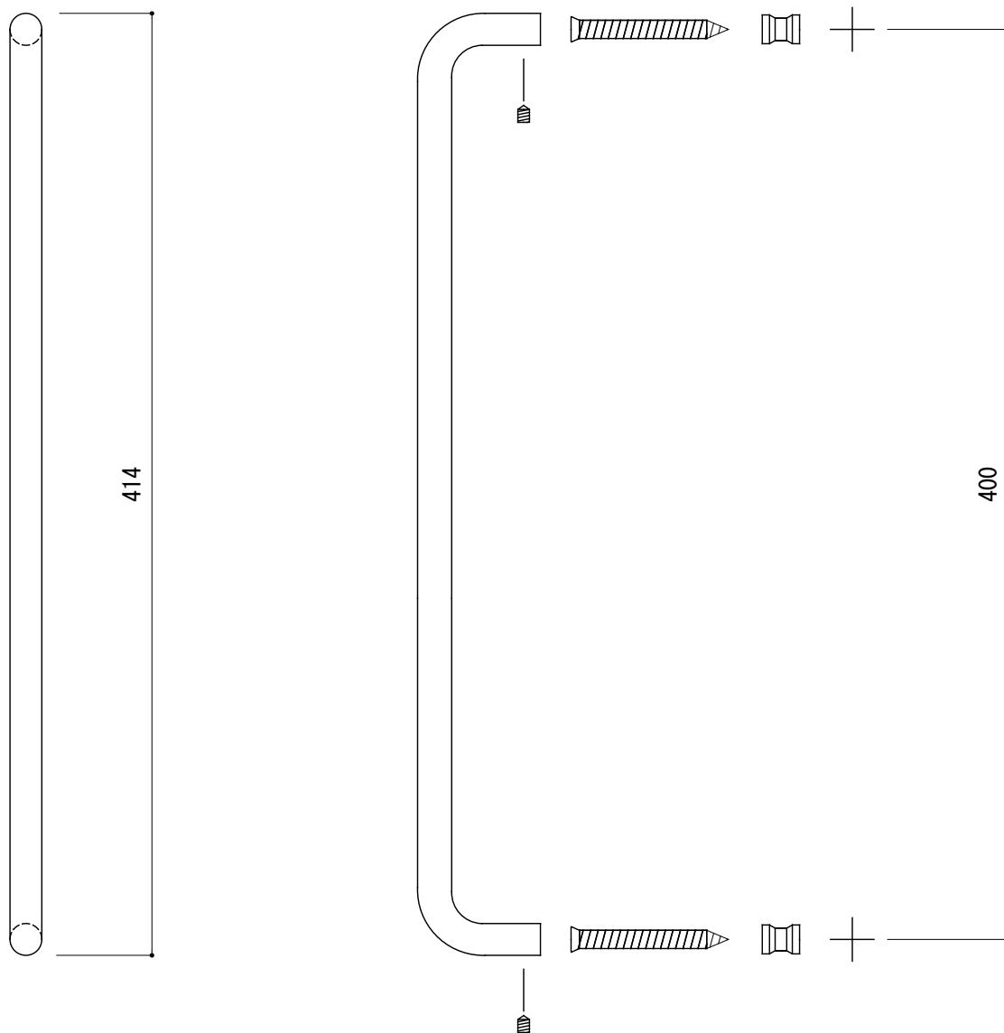
<切欠図>
